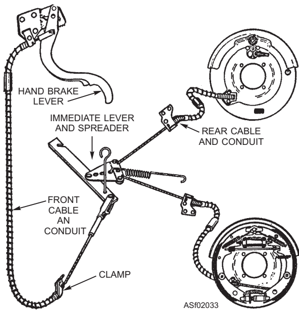
Figure 2-33.—Mechanical brake system—cables.
